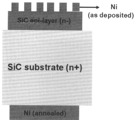
그림 5. SBD 구조. Fig. 5. SBD(Schottky Barrier Diode) structure.
