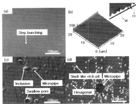
그림 3. 낮은 성장률(30 \mu\text{m}/\text{h} )을 가지는 SiC 에피택셜층의 표면 형상 (a) 광학현미경의 노말스키 모드 관찰 (b) AFM 결과, 스텝번칭의 높이는 약 100 nm (W와 H 스텝의 넓이와 높이를 표시한다.) (c) 약 100 \mu\text{m}/\text{h} 의 높은 성장률을 가지는 SiC 에피택셜층으로, 마이크로 파이프와 개재물 그리고 얇은 기공을 확인할 수 있다. (d) 에칭된 시편으로 (a)시편의 마이크로 파이프, 조개모양의 에피핏 그리고 육각형과 둥근 에치핏을 볼 수 있다. 450 ^{\circ}\text{C} KOH 용액으로 화학적 에칭을 하여 결함을 관찰하였다.
