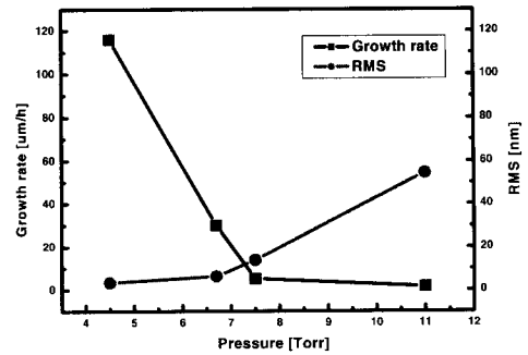
그림 4. 2000 ^{\circ}\text{C} 에서 성장 압력을 11에서 4.5 Torr로 줄였을 때, 성장률은 2에서 120 \mu\text{m}/\text{h} 였다. 그리고 높은 성장률은 낮은 성장 압력에서 얻을 수 있었으며, 이때 RMS값이 낮은 성장률 보다 낮았다.
