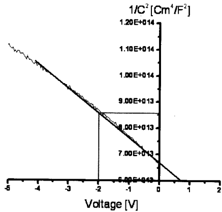
그림 6. SBD구조의 C-V 곡선, 전극의 직경은 180 \mu\text{m} , Vd 값은 0.7 V, N D 값은 1.4 x 10 18 cm -3 .
