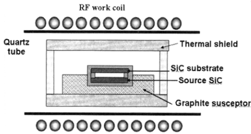
그림 1. 수평로 안의 내부 구조로서, 소스와 기판 사이의 거리를 1 mm로 유지 시켰다.
