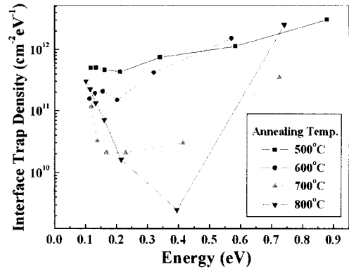
그림 6. 패시베이션 온도에 따른 Interface trap density. Fig. 6. Interface trap density as a function of passivation temperature.
