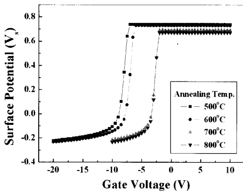
그림 5. 패시베이션 온도에 따른 Surface potential. Fig. 5. Surface potential as a function of passivation temperature.
