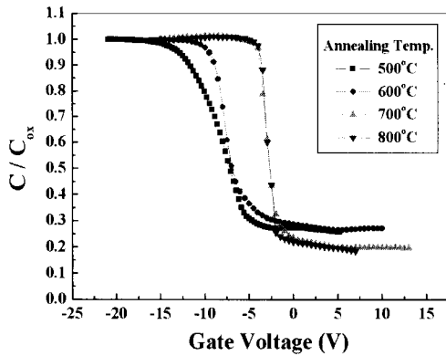
그림 4. 패시베이션 온도에 따른 Capacitance-voltage. Fig. 4. Capacitance-voltage as a function of passivation temperature.
