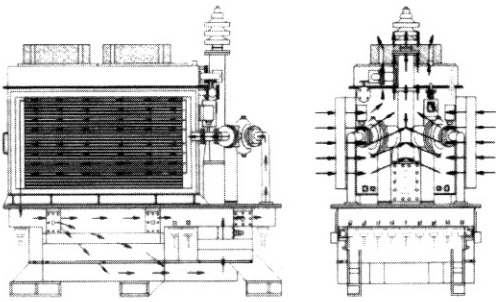
그림 1. 변압기의 오일 및 공기 흐름도.
