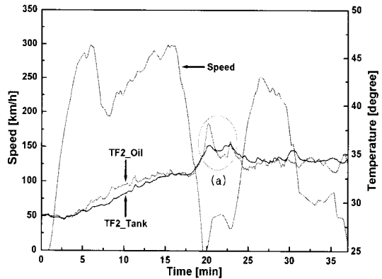
그림 6. 300 km/h에서의 변압기의 온도. Fig. 6. Transformer temperature running 300 km/h.
