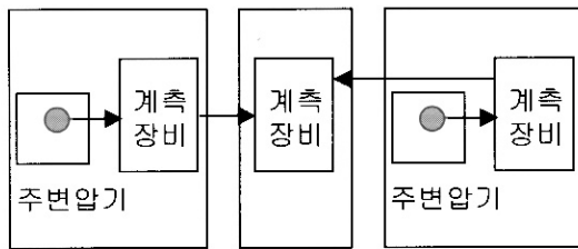
그림 3. 주변압기 온도측정 구성도. Fig. 3. Composition of temperature measurement for main transformer.
