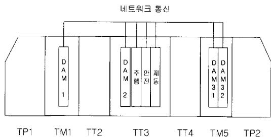
그림 2. 계측시스템의 구성도.
