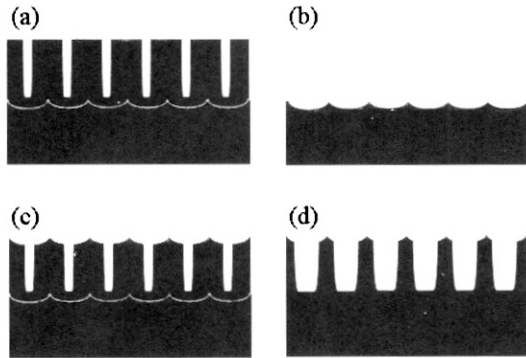
그림 1. 알루미늄 나노 템플레이트의 제작 과정도. (a) 1차 양극산화 후 다공성 알루미늄나층 형성 (b) 다공성 알루미늄나층 제거 (c) 2차양극산화 후 정렬된 다공성 알루미늄나층 (d) 기공 확장 과정
