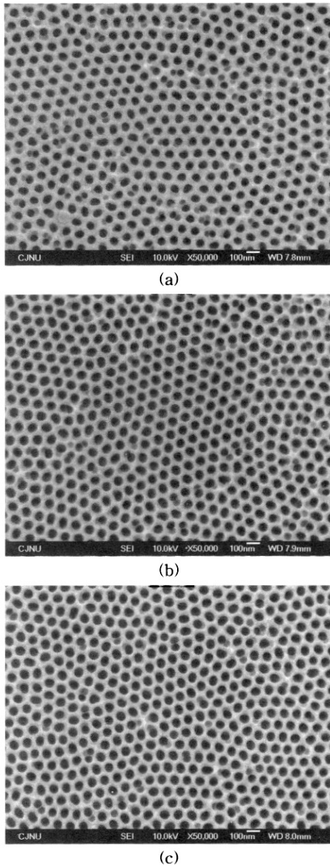
그림 6. 열처리 에너지원과 시간에 대한 AAO 템플레이트의 FE-SEM이미지.
