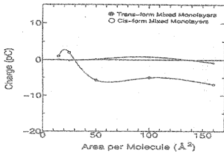
그림 7. 6Az5PVA와 5CB 혼합막의 전하량 비교. Fig. 7. Compare of charge amount with 6Az5PVA and 5CB mixed molecule.
