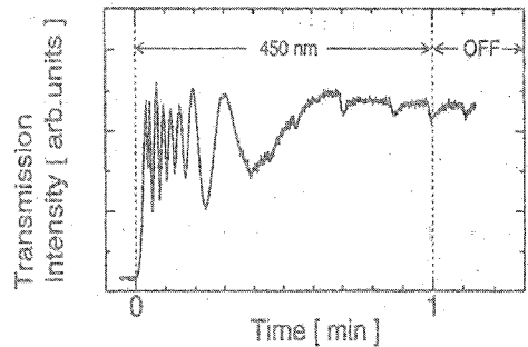
(b) 트랜스체 → 시스체
