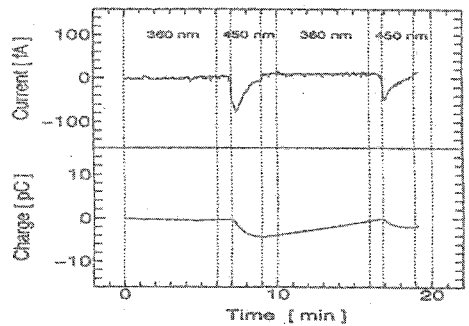
(b) 시스 전개체
