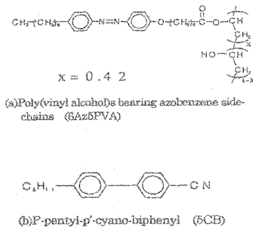
그림 1. 분자 구조. Fig. 1. Molecular structure.
