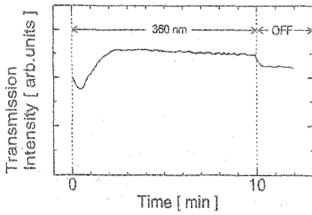
(a) 트랜스체 → 시스체
