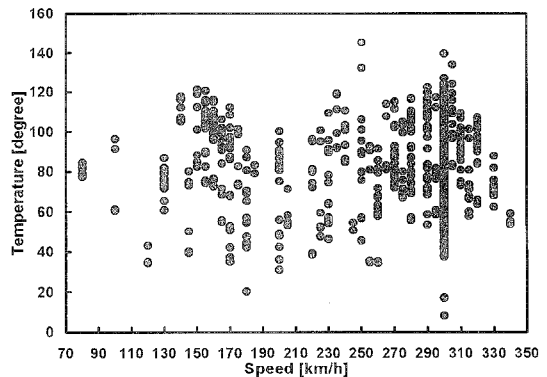
그림 8. 속도별 전동기 온도.
