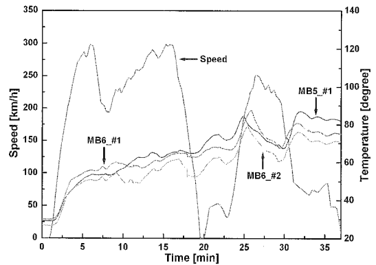
그림 5. 300 km/h 속도에서의 전동기 온도. Fig. 5. Traction motor temperature running 300 km/h.
