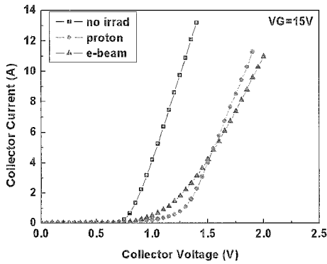
그림 3. IGBT 소자의 컬렉터 포화 전류 특성 (VG=15 V).
