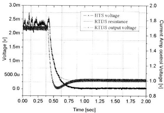
그림 9. 고장 소멸 후, 피드백 전압의 변화. Fig. 9. After fault extinction, change of feedback voltage level according to the current which flows into HTS wire.
