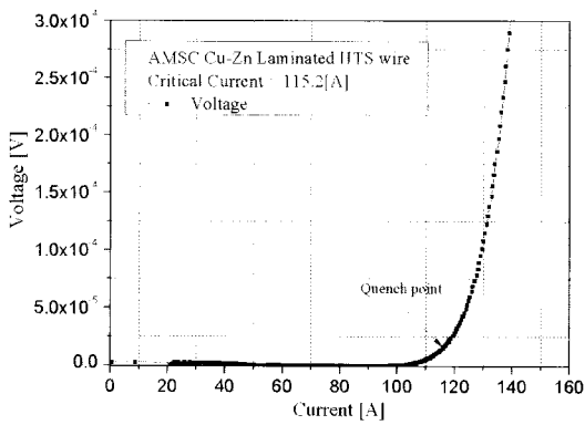
그림 3. 실험에 사용된 Bi-2223 HTS wire의 V-I 그래프. Fig. 3. V-I Curve of the Bi-2223 HTS wire used in experiment.
