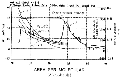
그림 6. 쌍극자 모멘트를 변화 시켰을 때의 시뮬레이션 결과.
