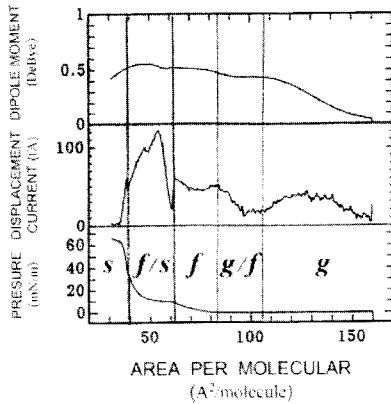
그림 4. 수면상 성막 물질의 \pi -A, \pi -I, \pi -D의 관계. Fig. 4. \pi -A, \pi -I, and \pi -D isotherms of L-film on water surface.
