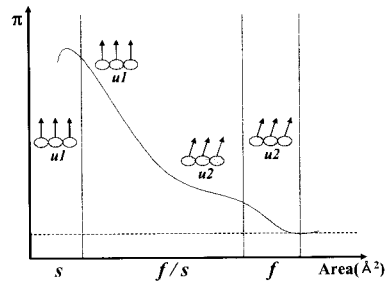
그림 5. 고체상태, 액체/고체 혼재 상태, 액체 상태의 단분자 상태와 쌍극자 모멘트의 가정. Fig. 5. Assumption of dipole moment and monolayer, fluid, liquid/fluid and solid state.
