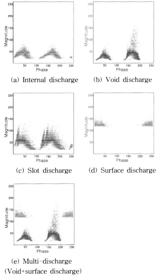
그림 1. 개개의 방전원과 다중방전원의 PD패턴.
