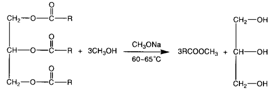
그림 1. 대두유와 메탄올의 에스테르화 반응.
