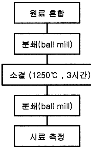
그림 1. 형광체 합성의 순서도. Fig. 1. Flow chart of phosphor synthesis.
