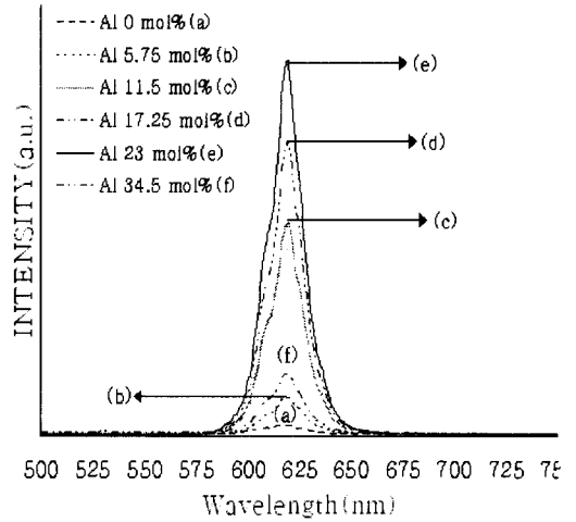
그림 5. Al 3+ 의 몰 변화에 따른 SrTiO 3 :Al,Pr의 광여기 발광 스펙트럼. Fig. 5. PL emission spectra of SrTiO 3 :Al, Pr with various molar ratios of Al 3+ under the 365 nm excitation at room temperature.
