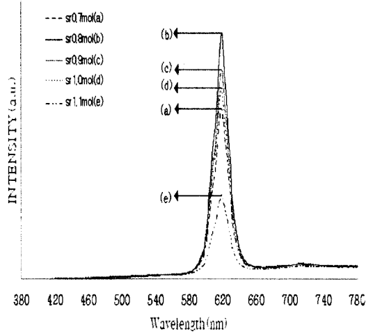
그림 8. 1000 V, 100 \mu A/cm^2 조건하에서 Sr^{2+} 의 몰 변화에 따른 SrTiO_3:Al,Pr 의 음극선 여기 발광 스펙트럼. Fig. 8. CL emission spectra of SrTiO_3:Al,Pr with various molar ratios of Sr^{2+} under the 1000 V, 100 \mu A/cm^2 condition.
