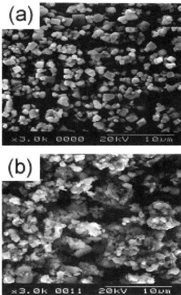
그림 4. SrTiO 3 :Al,Pr의 SEM 이미지. (a)Al 0 mol%, (b) Al 23mol% Fig. 4. SEM images of SrTiO 3 :Al,Pr. (a)Al 0 mol% and (b) Al 23 mol%
