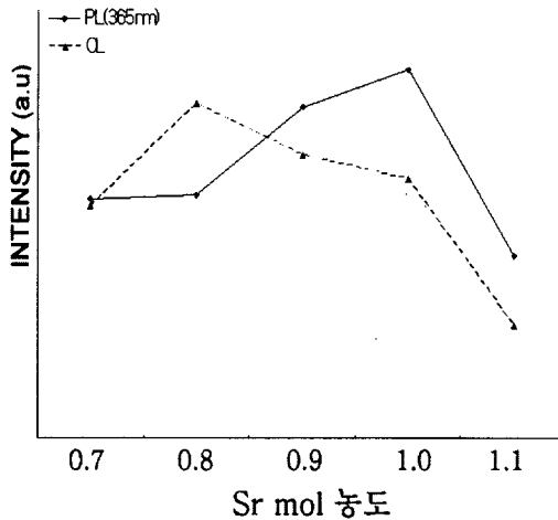
그림 10. Sr^{2+} 이온의 몰 변화에 따른 SrTiO_3:Al,Pr 의 광 여기 발광과 음극선 여기 발광의 세기 비교.
