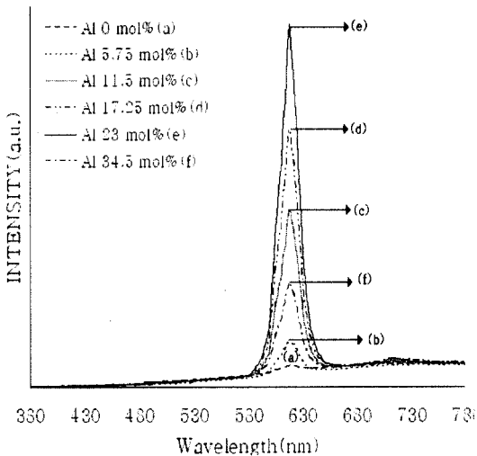
그림 7. 1000 V, 100 \mu A/cm^2 조건하에서 Al^{3+} 의 몰 변화에 따른 SrTiO_3:Al,Pr 의 음극선 여기 발광 스펙트럼. Fig. 7. CL emission spectra of SrTiO_3:Al,Pr with various molar ratios of Al^{3+} under the 1000 V, 100 \mu A/cm^2 condition.
