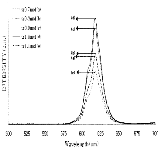
그림 6. Sr^{2+} 의 몰 변화에 따른 SrTiO_3:Al,Pr 의 여기 발광 스펙트럼. Fig. 6. PL emission spectra of SrTiO_3:Al,Pr with various molar ratios of Sr^{2+} under the 365 nm excitation at room temperature.
