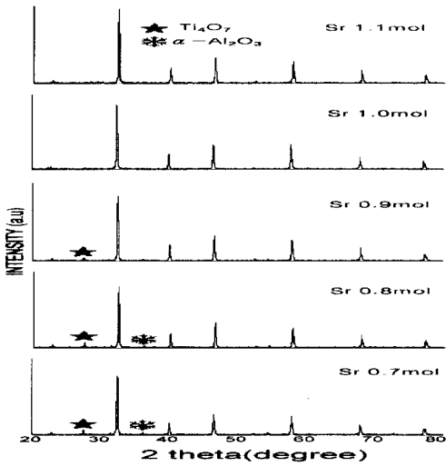
그림 3. SrTiO 3 :Al,Pr의 Sr 2+ 의 다양한 몰 변화에 따른 XRD 패턴. Fig. 3. XRD patterns of SrTiO 3 :Al,Pr with various molar ratios of Sr 2+ .
