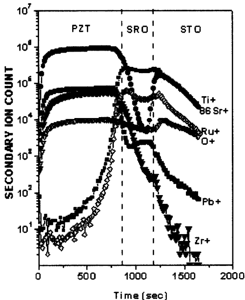
그림 4. 650 °C에서 증착된 PZT(56 nm)박막의 SIMS depth-profile.
