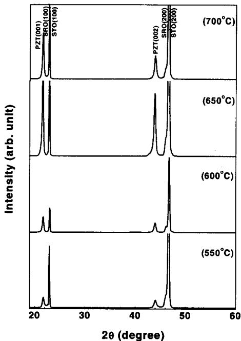
그림 2. 증착 온도에 따른 PZT 박막의 XRD 패턴. Fig. 2. XRD patterns of 56 nm thick-PZT thin films grown at various temperatures.
