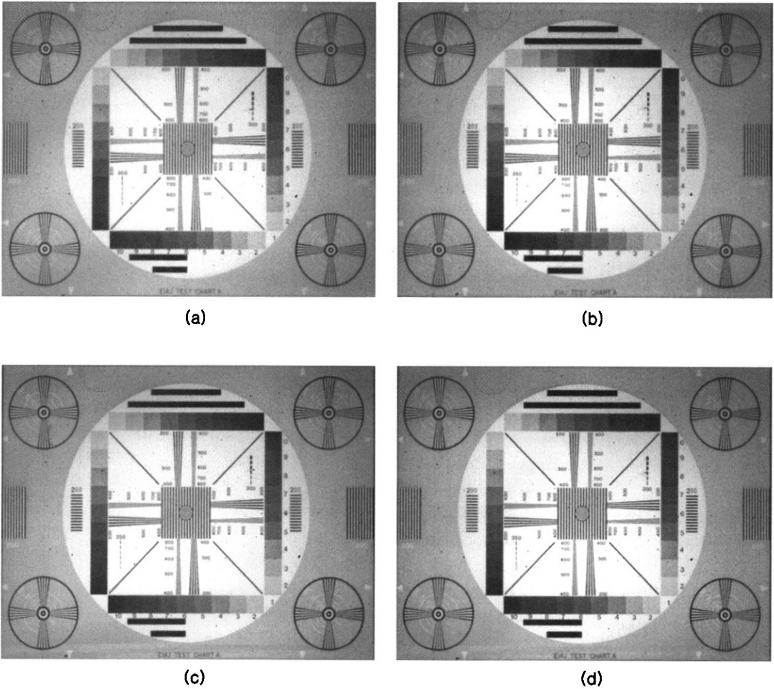
그림 6. EIAJ 도표 촬영 사진. HOLF의 위상차는 각각 (a) \pi , (b) 0.9 \pi , (c) 0.8 \pi , (d) 0.7 \pi 이다. Fig. 6. Images of EIAJ chart. The phase differences of HOLF: (a) \pi , (b) 0.9 \pi , (c) 0.8 \pi , (d) 0.7 \pi .
