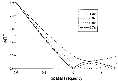
그림 2. 설계된 HOLF의 위상차를 변화시키며 계산한 MTF 그래프.
