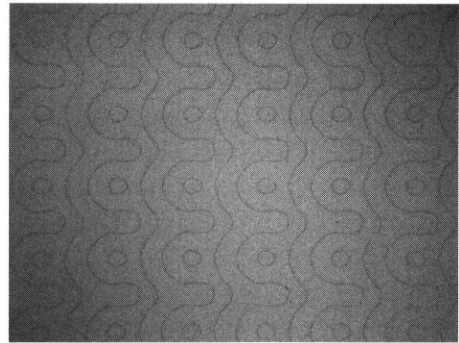
그림 3. 제작된 21-빔 HOLF의 현미경 사진. 홀로그램의 주기는 120 \mu\text{m} 이다. Fig. 3. The photomicrography of 21-beam HOLF. The period of HOLF is 120 \mu\text{m} .
