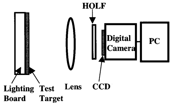
그림 4. HOLF 실장 실험을 위한 장치도. Fig. 4. Experimental setup to take pictures of test charts by a camera with HOLF.
