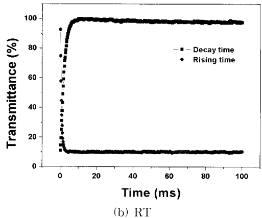
그림 6. 새로운 HTOCB 셀의 전압투과율 및 응답 특성.
