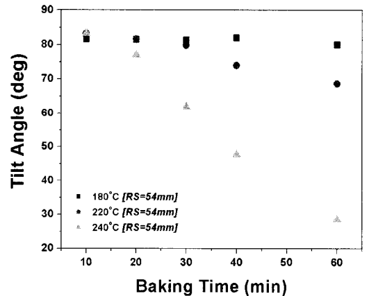
그림 4. 정(+)의 액정을 이용하여 수직 폴리이미드 표면에서의 소성 온도 및 시간에 따른 네마틱 액정의 프리틸트각의 발생.
