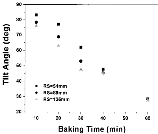
그림 5. 정(+)의 액정을 이용하여 수직 폴리이미드 표면에서의 소성 온도 및 리빙강도에 따른 네마틱 액정의 프리틸트각의 발생. Fig. 5. Generation of tilt angle in NLC on the homeotropic polyimide surface as a function of hotplate temperature and rubbing strength using positive type NLC.
