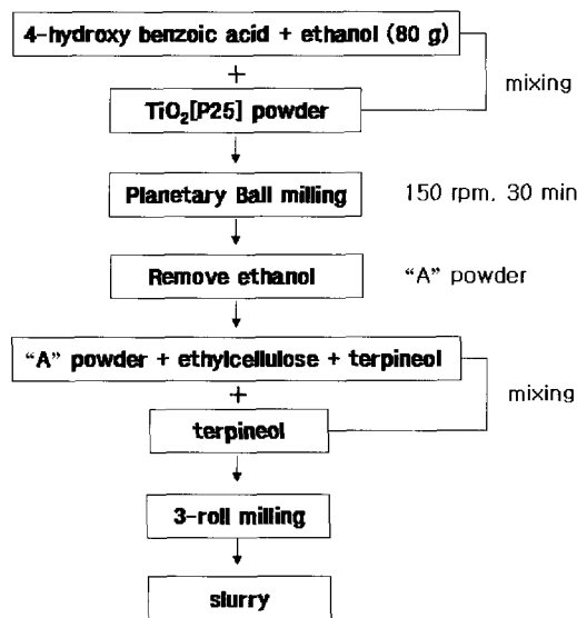
그림 1. 슬러리 제조 공정도.
