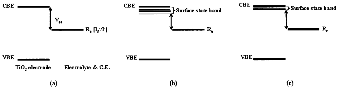
그림 5. \text{TiO}_2 전극표면에서의 에너지 준위 모식도.
