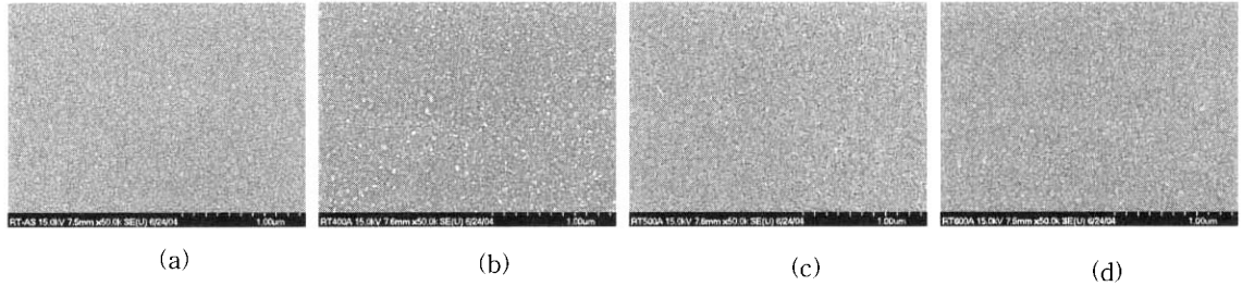
그림 1. 공기 중에서 다양한 온도 조건에 따라 6시간 열처리한 NiCr의 표면 및 단면 FESEM 사진; (a) 증착 후, (b) 400 °C, (c) 500 °C, (d) 600 °C.
