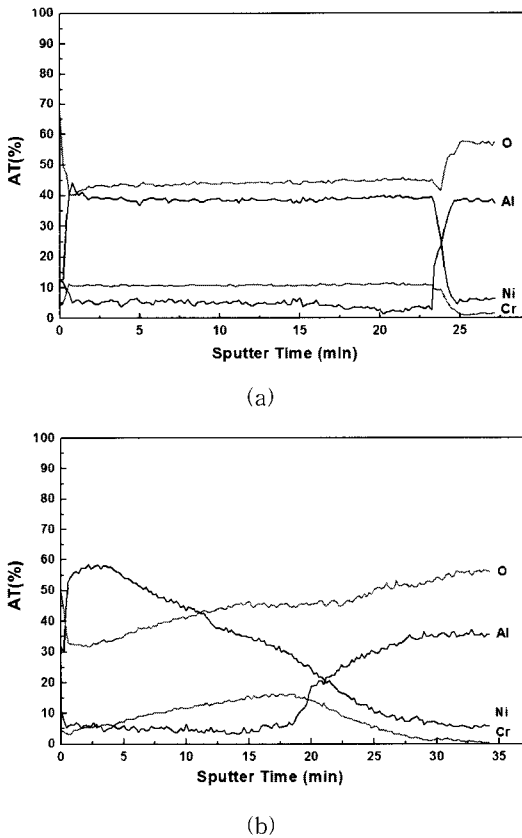
그림 3. NiCr 박막의 깊이에 따른 조성분석 (a) 열처리 전 시편 (b) 500 °C에서 수소 분위기로 6시간동안 열처리한 시편.
