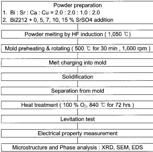
그림 1. 실험 공정도.
