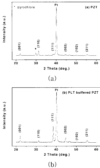
그림 3. (a) PZT (b) PLT buffer가 사용된 PZT 박막의 XRD pattern.
