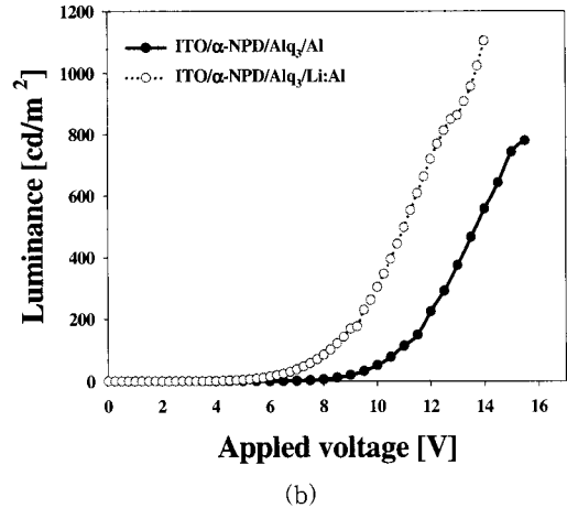
그림 3. 음극 변화에 따른 OLEDs의 (a) 전압-전류밀도, (b) 전압-휘도 특성. Fig. 3. (a) Voltage vs. current density and (b) voltage vs. luminance characteristics of OLEDs at different cathode.
