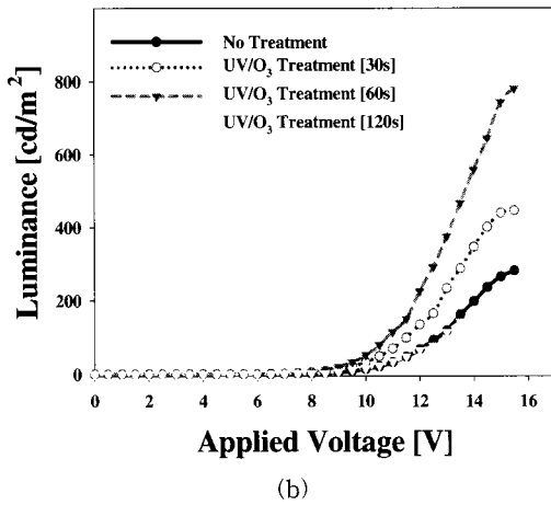
그림 2. UV/O 3 처리 시간에 따른 OLEDs의 (a) 전압-전류밀도 특성, (b) 전압-휘도 특성. Fig. 2. (a) Voltage vs. current density and (b) voltage vs. luminance characteristics of OLEDs at different UV/O 3 treatment time.
