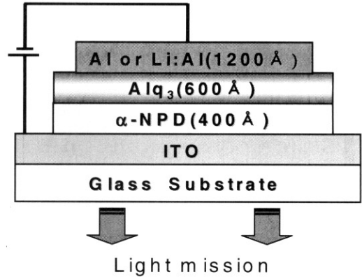
그림 1. OLEDs의 구조.
