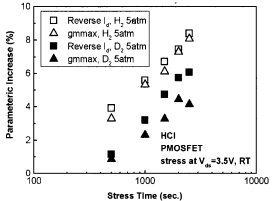
그림 5. PMOSFET의 HCl 열화(상온) 특성.
