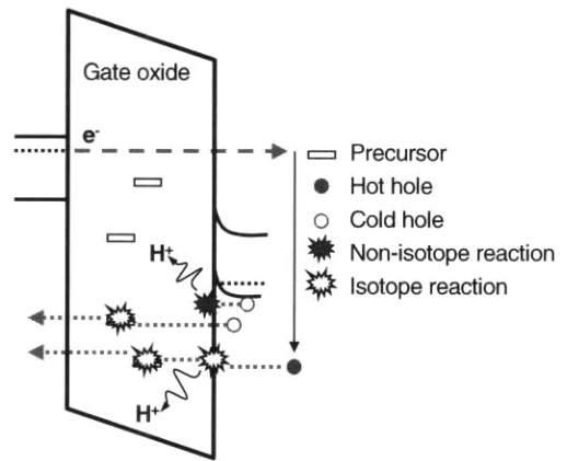
그림 8. 게이트 산화막내에서 발생하는 결합. Fig. 8. Illustration of the generation of defects in gate oxide film.
