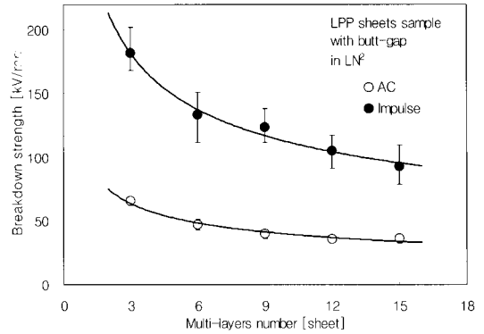
그림 3. LPP 시료의 적층 수에 따른 절연과피 전계. Fig. 3. Breakdown strength of LPP sheets sample on multi-layered number.
