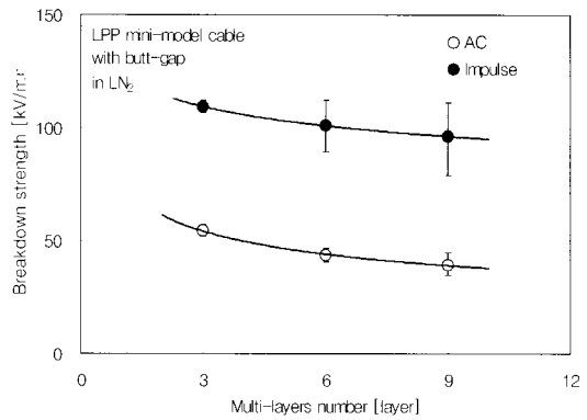
그림 6. 미니모델 케이블의 적층 수에 따른 절연 파괴 전계.
