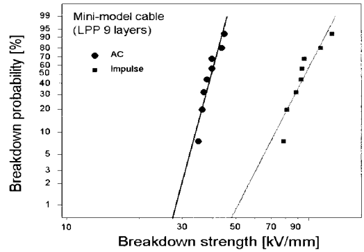
그림 7. 미니모델 케이블의 AC 및 임펄스 절연 파괴 전계의 와이불 분포도.
