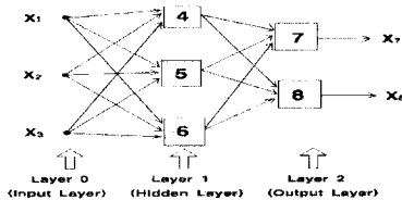
그림 3. MLP-BP의 구조. Fig. 3. Architecture of MLP-BP.
