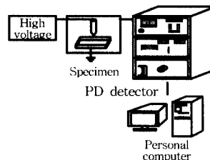
그림 2. PD측정시스템의 블록도.
