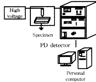
그림 2. PD 측정시스템의 블록도.
