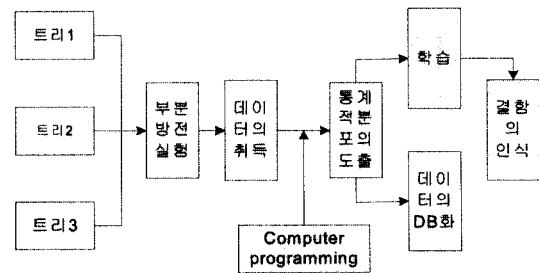
그림 3. PD데이터의 처리흐름도.
