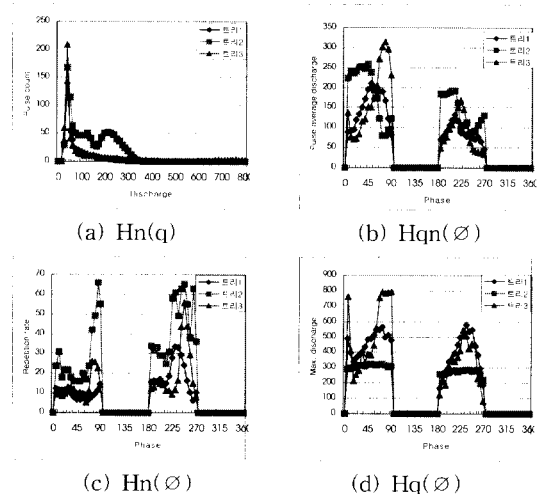
그림 5. 트리방전의 통계적 분포.
