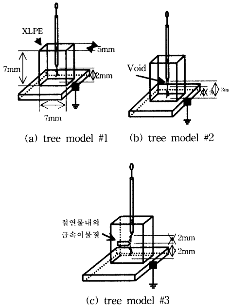
그림 1. 세 가지 경우의 시편형상.
