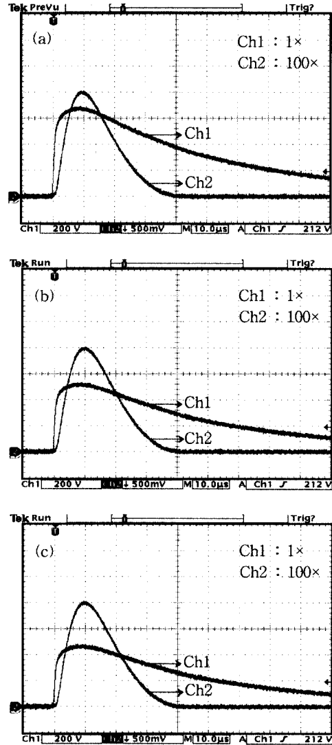
그림 4. 소결온도에 따른 ZPCCE계 바리스터의 제한전압특성; (a) 1335°C, (b) 1340°C, (c) 1345°C.
