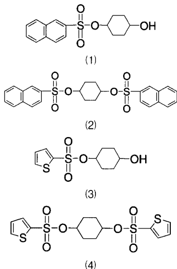
그림 1. 산 증식제의 구조. Fig. 1. Structures of acid amplifiers.
