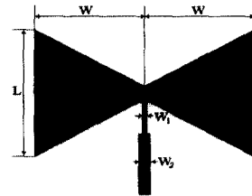
그림 3. 광대역 초전도 안테나의 단일 소자 패턴.
