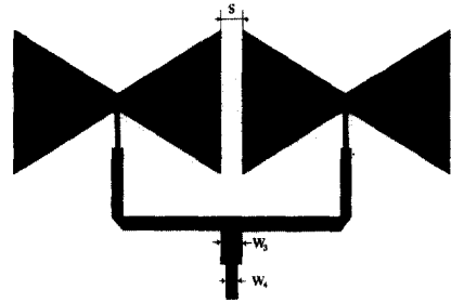
그림 2. \epsilon_r=9.6 , t = 0.5 mm인 MgO 기관 위에 50 \Omega 급전선으로 급전되는 광대역 초전도 안테나의 Layout.
