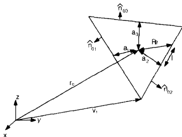
그림 1. 삼각형에서 표면적분 계산을 위한 기하학적 양.
