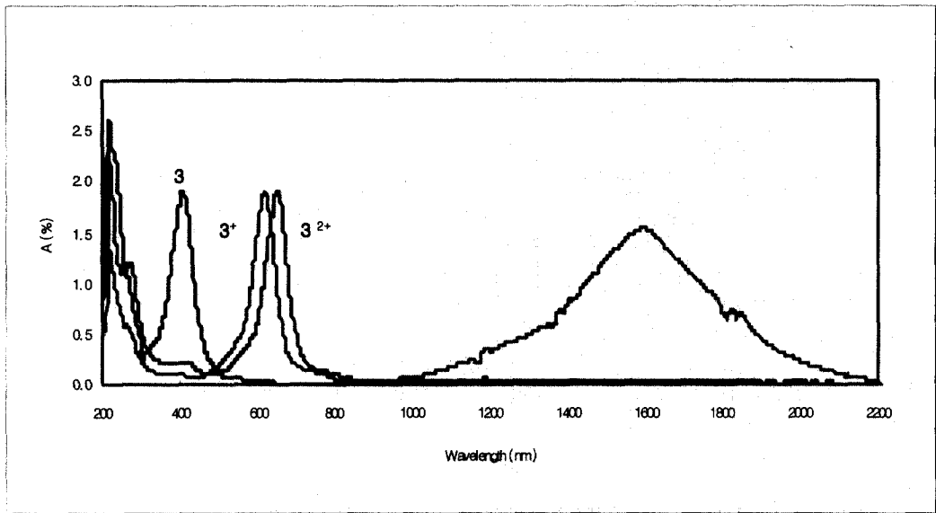
그림 5. 화합물 3의 중성, cation, dication에 대한 UV/Vis-Near IR.
