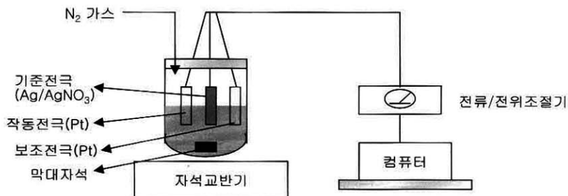
그림 3. 순환 전위 전류 실험.
