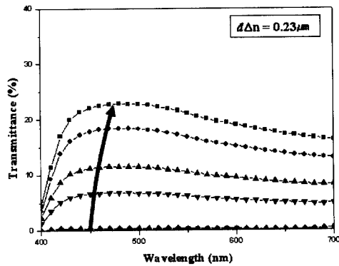
그림 10. d\Delta n 이 0.23 \mu m 인 IPS 셀의 계조별 투과율의 파장 의존성.
