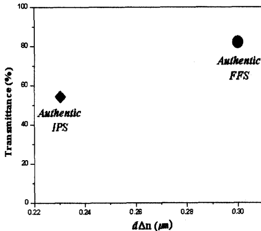
그림 15. Authentic-color IPS 셀과 FFS 셀의 최대 투과율과 d\Delta n .
