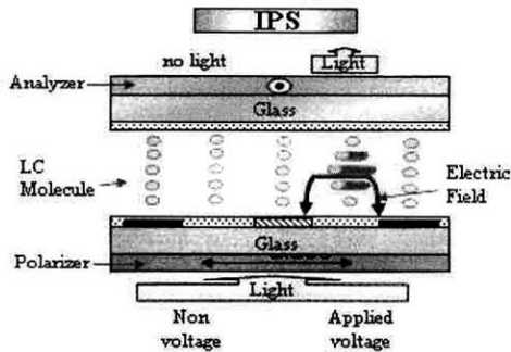
그림 5. IPS 셀의 셀 구조와 동작원리. Fig. 5. Cell structure and switching principle of a IPS cell.
