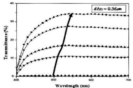
그림 8. d\Delta n 이 0.36 \mu\text{m} 인 FFS 셀의 계조별 투과율의 파장 의존성.
