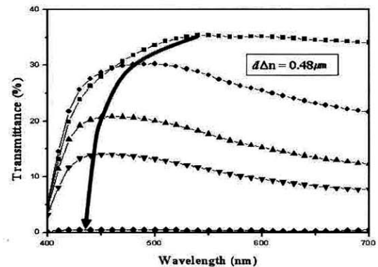
그림 2. d\Delta n 이 0.48 \mu\text{m} 인 TN 셀의 계조별 투과율의 파장 의존성.
