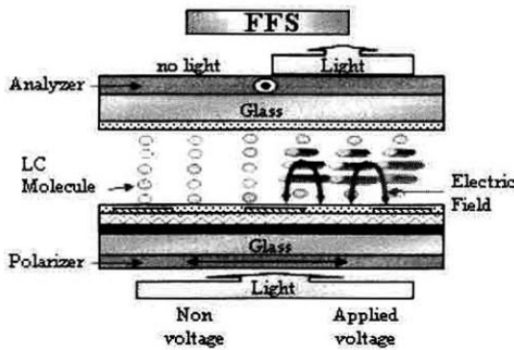
그림 6. FFS 셀의 셀 구조와 동작원리. Fig. 6. Cell structure and switching principle of a FFS cell.
