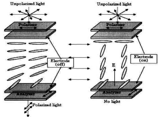
그림 1. TN 셀의 셀 구조와 동작 원리.
