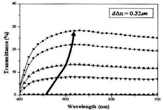
그림 7. d\Delta n 이 0.32 \mu\text{m} 인 IPS 셀의 계조별 투과율의 파장 의존성.
