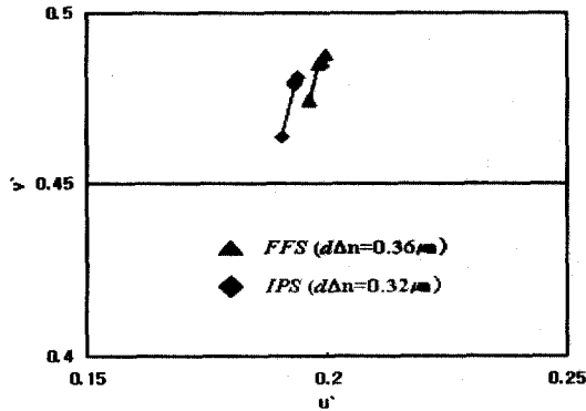
그림 9. d\Delta n 이 0.36 \mu\text{m} 인 FFS 셀과 0.32 \mu\text{m} 인 IPS 셀의 색끌림.
