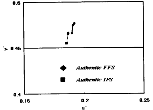
그림 12. Authentic-color IPS 셀과 FFS 셀의 색갈림.
