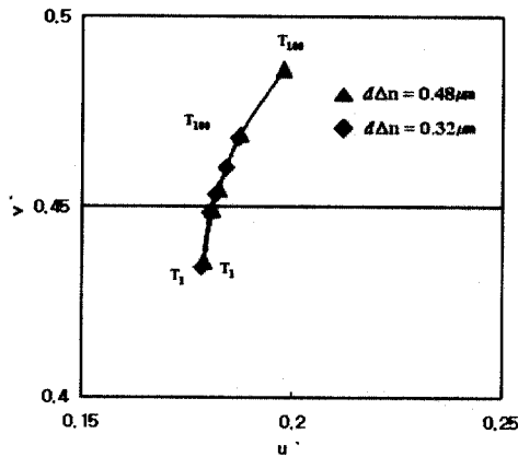
그림 4. d\Delta n 이 0.48 \mu\text{m} 과 0.32 \mu\text{m} 인 TN 셀들의 색궤. Fig. 4. Color tracking of TN cell when d\Delta n values are 0.48 \mu\text{m} and 0.32 \mu\text{m} .
