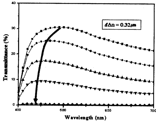
그림 3. d\Delta n 이 0.32 \mu\text{m} 인 TN 셀의 계조별 투과율의 파장 의존성. Fig. 3. Wavelength dependent-transmittance of each gray scale in the TN cell of which the d\Delta n value is 0.32 \mu\text{m} .
