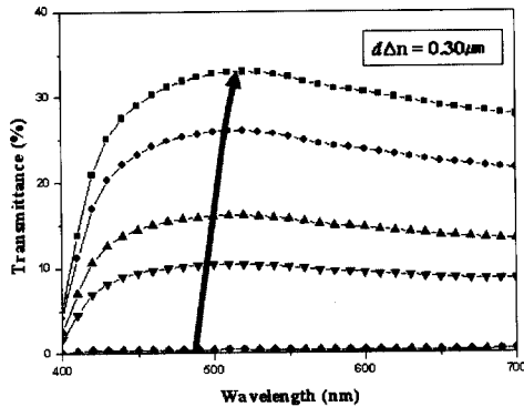
그림 11. d\Delta n 이 0.30 \mu m 인 FFS 셀의 계조별 투과율의 파장 의존성.
