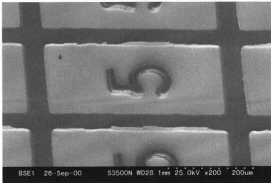
그림 3. 미소담체의 SEM 이미지. Fig. 3. SEM images of the particle.
