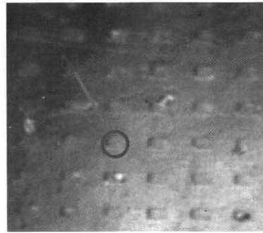
그림 4. Ni 도트의 SEM 이미지. Cr/Au/Ni 층의 구조.
