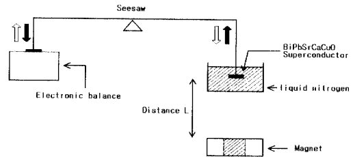
그림 4. Seesaw에 의한 자기력 측정 장치. Fig. 4. Schematic diagram of the apparatus for the magnetic force measurement by seesaw.
