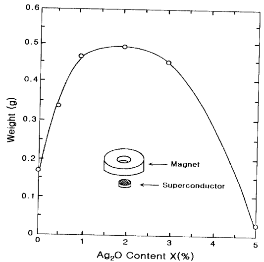
그림 2. 초전도 시료의 중량변화.
