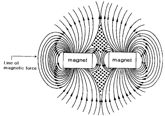
그림 6. Toroidal 자석의 자력선 분포 모델.
