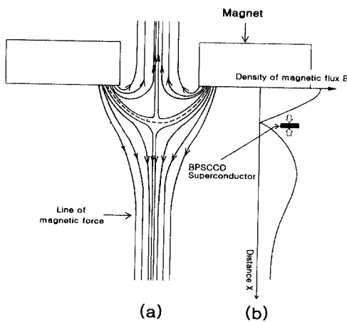
그림 10. 자력선 분포와 자속 밀도 분포.
