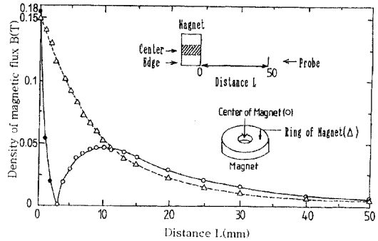
그림 9. Toroidal 자석의 자속 밀도 분포. Fig. 9. Distribution of magnetic flux density arising from the toroidal magnet.
