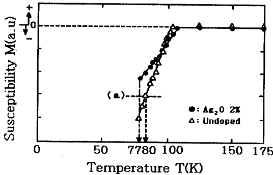
그림 3. 직류자화율의 온도의존성. Fig. 3. Temperature dependence of the DC susceptibility.
