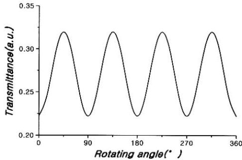
그림 3. Twist 배열된 액정 셀을 직교된 편광판 사이에서 회전시켰을 때의 투과율 변화.
