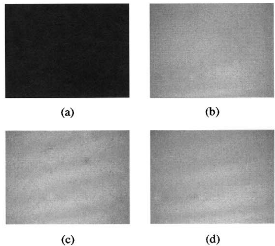
그림 2. OCS 셀 관찰 사진 : (a) 흑 상태, (b) 명 상태, (c)와 (d)는 (b)를 45°와 90°로 회전.
