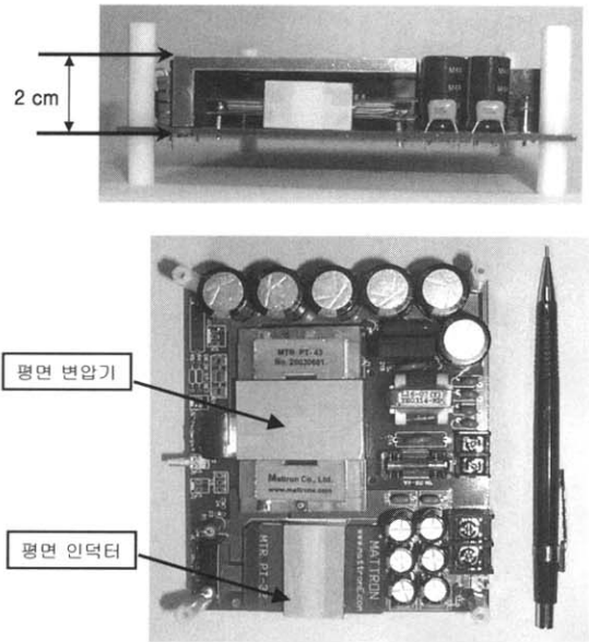
그림 8. 평면 변압기가 채용된 파워드 컨버터. Fig. 8. Forward converter equipped with planar transformer.
