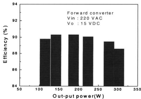
그림 10. 컨버터의 효율. Fig. 10. Efficiency of converter.
