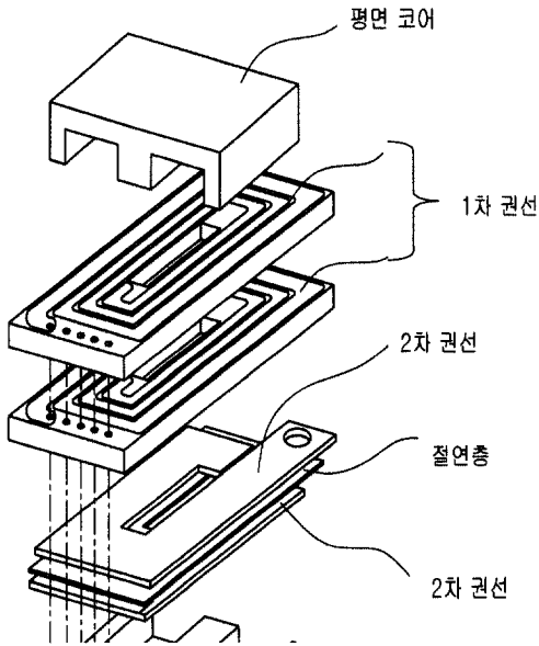
그림 1. 평면 변압기의 구조. Fig. 1. Structure of planar transformer.
