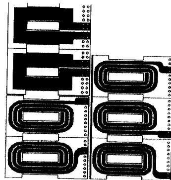
그림 3. 평면 변압기 권선 패턴.
