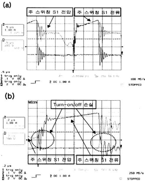
그림 9. 주 스위칭소자의(S) 전압 및 전류 파형: (a) 한 주기, (b) 확대 파형(360 W). Fig. 9. Voltage and current wave of switching device at 360 W : (a) one cycle, (b) magnification wave.
