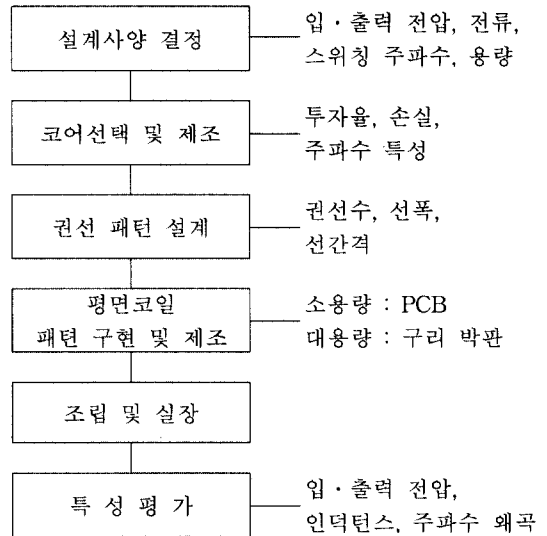
그림 2. 평면 변압기 제조 공정. Fig. 2. Manufacturing process for planar transformer.
