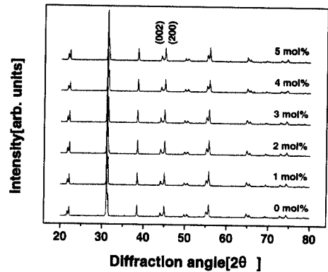
그림 3. BiFeO 3 치환에 따른 X선 회절 패턴(950 °C).
