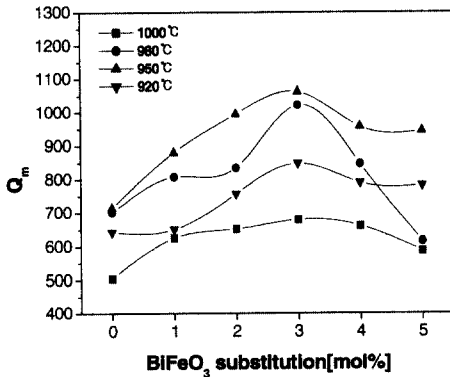
그림 5. BiFeO 3 치환에 따른 기계적품질계수. Fig. 5. Mechanical quality factor with BiFeO 3 substitution.
