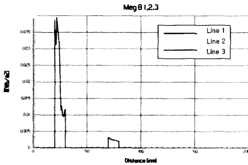
그림 6. 방전튜브 내부의 x축상의 거리에 대한 자속밀도 분포. Fig. 6. Distribution of magnetic flux density according to distance on the X-axis inside of tube.
