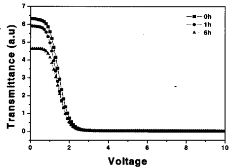
그림 2. 폴리이미드 표면을 이용한 3종류의 TN 셀의 V-T 곡선.
