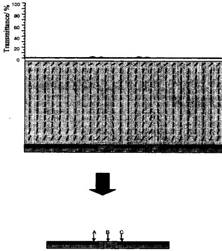
그림 2. 전극 위치별 액정 방향자 분포도 및 투과율. 인가전압: 화소전극 (1V), data bus line (1V), 공통 전극 (6V).
