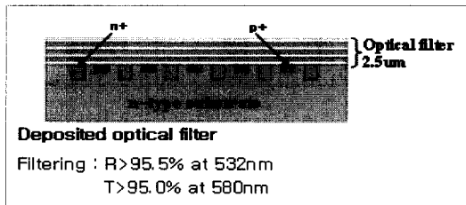
그림 8. 광학 필터가 증착된 광센서.
