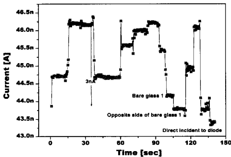
그림 12. LED 광원을 이용한 형광 검출. Fig. 12. Fluorescence detection using LED.
