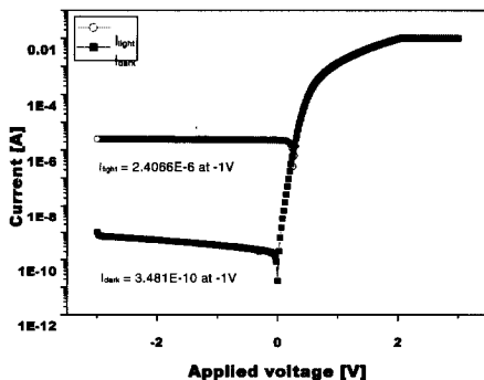
그림 9. 광학 필터가 증착된 광센서의 I-V 특성.
