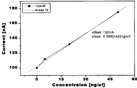
그림 11. 집적화된 LOC에서의 형광 측정. Fig. 11. Fluorescence detection in integrated LOC.
