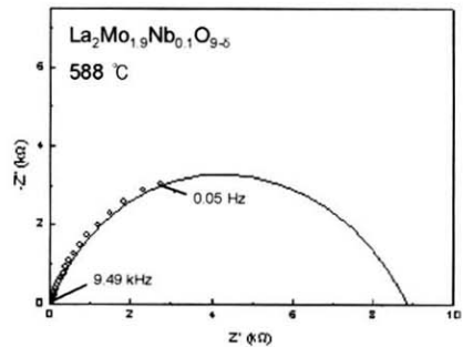
그림 4. 공기중 588°C에서 \text{La}_2\text{Mo}_{1.9}\text{Nb}_{0.1}\text{O}_{9.6} 의 복소 임피던스 스펙트럼(o; 측정값, 실선; 계산값).
