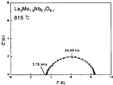
그림 5. 공기중 815°C에서 \text{La}_2\text{Mo}_{1.9}\text{Nb}_{0.1}\text{O}_{9.6} 의 복소임피던스 스펙트럼( \circ ; 측정값, 실선; 계산값).
