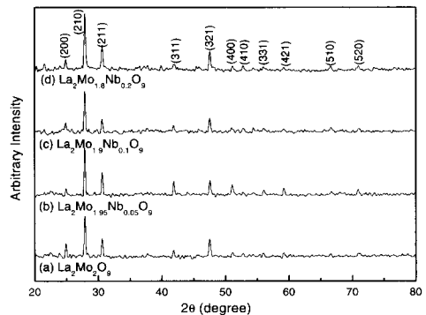
그림 1. La 2 Mo 2-x Nb x O 9 의 X선 회절도.
