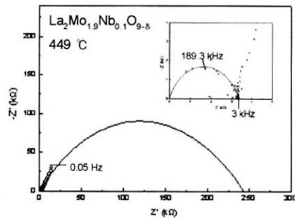
그림 3. 공기중 449°C에서 \text{La}_2\text{Mo}_{1.9}\text{Nb}_{0.1}\text{O}_{9.6} 의 복소 임피던스 스펙트럼(o; 측정값, 실선; 계산값).
