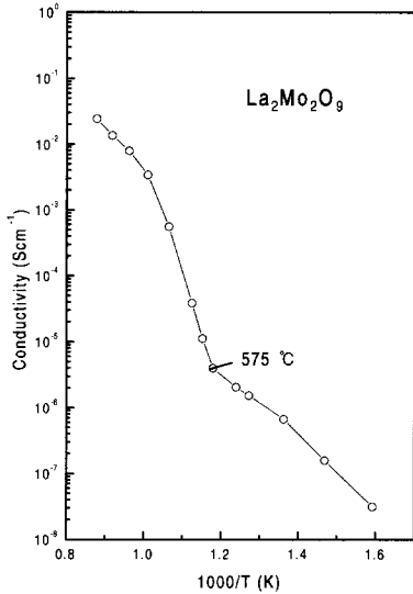
그림 6. \text{La}_2\text{Mo}_2\text{O}_9 의 전기전도도의 아레니우스 플롯.
