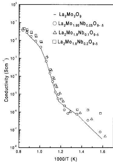
그림 7. \text{La}_2\text{Mo}_{2-x}\text{Nb}_x\text{O}_{9-\delta} 의 전기전도도의 아레니우스 플롯.
