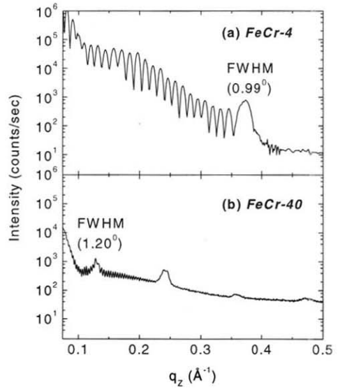
그림 2. Cr층의 두께가 서로 다른 (a) FeCr-4 다층박막과 (b) FeCr-40 다층박막에서 얻어진 x-선 반사법 곡선들. Fig. 2. X-ray reflectivity profiles obtained on (a) the monatomic FeCr-4 and (b) FeCr-40 multilayers with different Cr-layer thickness.
