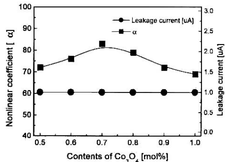
그림 5. 시편의 비직선계수와 누설전류. Fig. 5. \alpha and I_i of ZnO varistors with variation of \text{Co}_3\text{O}_4 .
