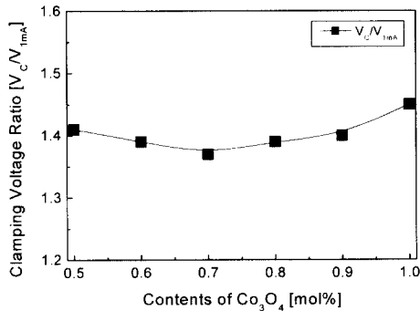
그림 6. 시편의 제한전압비.
