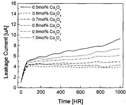
그림 8. 시험의 고온부하시험 결과.
