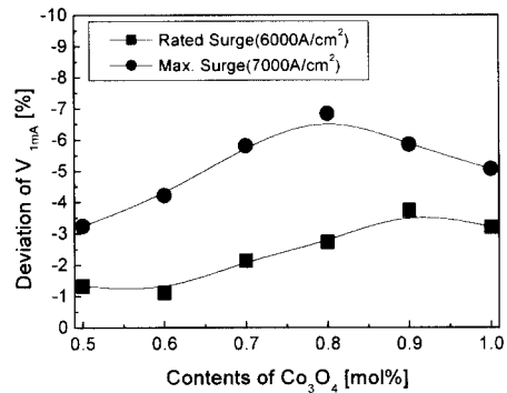
그림 7. 시편의 서지내량 측정 결과.
