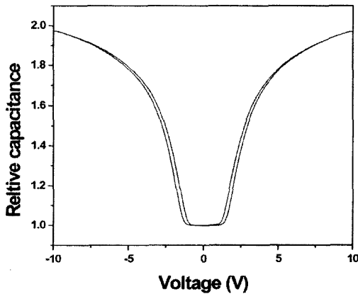
그림 9. 광폴리머 표면을 이용한 광배향 TN-LCD의 C-V 특성.
