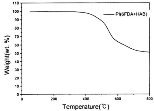
그림 4. 광폴리머의 TGA 특성. Fig. 4. TGA characteristics of photopolymer.
