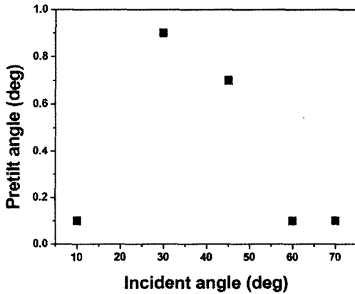
그림 6. 광폴리머 표면에 편광된 UV를 조사시의 조사각도에 따른 네마틱액정의 프리틸트각의 발생.
