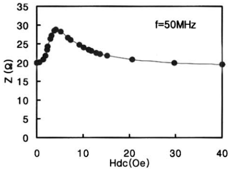
그림 7. 직류 외부자기 변화에 따른 MI소자의 임피던스.
