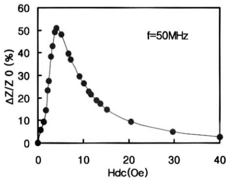
그림 8. 직류 외부자기 변화에 따른 MI소자의 임피던스 변화율.
