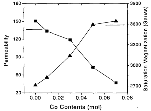
그림 5. Co 첨가량에 따른 포화자속 밀도와 투자율 변화.
