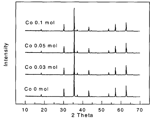
그림 1. Ni_{0.8-x}Zn_{0.2}Co_xFe_2O_4 의 Co 첨가량에 따른 X-선 회절분석 결과.
