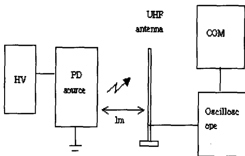
그림 2. 실험 장치에 대한 블록나이어그램.
