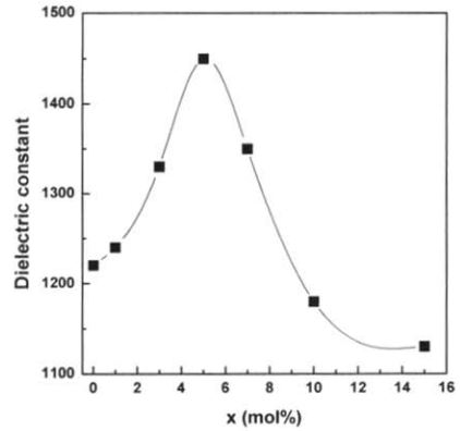
그림 4. PAN 첨가량에 따른 xPAN-(1-x)PZT 박막의 유전상수. Fig. 4. Dielectric constant of xPAN-(1-x)PZT thin films as a function of x.
