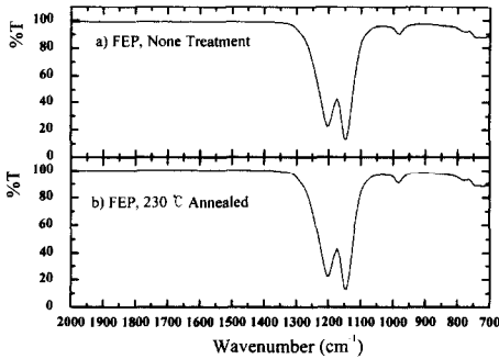
그림 5. 열처리 전 FEP와 230 °C에서 열처리 된 FEP의 FT-IR 특성 곡선. Fig. 5. FT-IR spectra of FEP films before(a) and after annealing(b).
