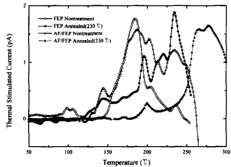
그림 3. 음극 코로나 하전후 230 °C에서 열처리된 FEP 및 AF/FEP 이중 필름과 열처리 전시편의 TSC 특성 곡선
