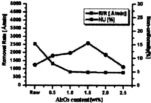
그림 4. 알루미늄 연마제 함량에 따른 연마율과 비균일도 관계.
