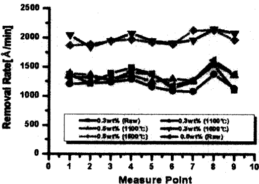
그림 5. 열처리한 알루미늄 연마제의 연마율 특성.
