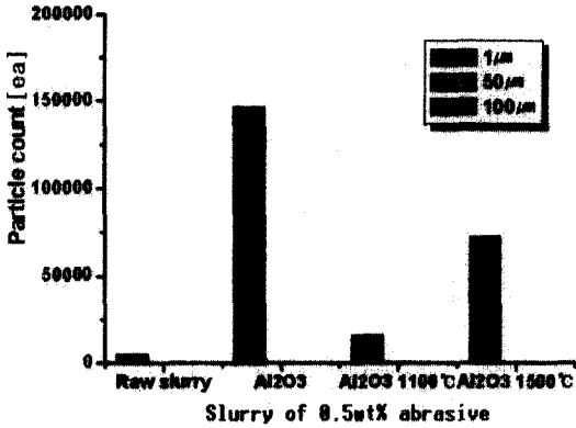
그림 7. 슬러리의 입자수.
