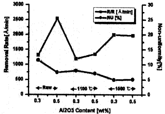
그림 6. 열처리한 알루미늄 연마제의 연마율과 비균일도 특성.
