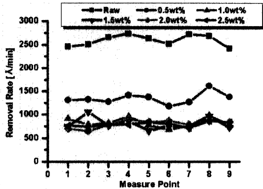
그림 2. 알루미나 연마제 첨가 함량에 따른 연마율 비교.
