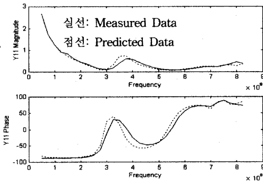
그림 7. 테스트 구조 3-L의 측정된 Y11과 예측된 Y11.
