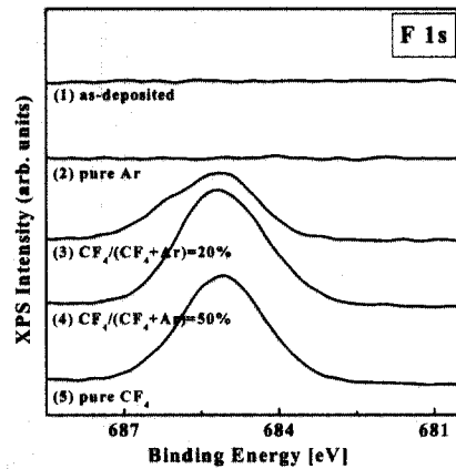
그림 8. CF 4 /Ar 혼합비에 따라 식각된 PST 박막의 표면에서 F 피크의 XPS narrow scan 스펙트럼.
